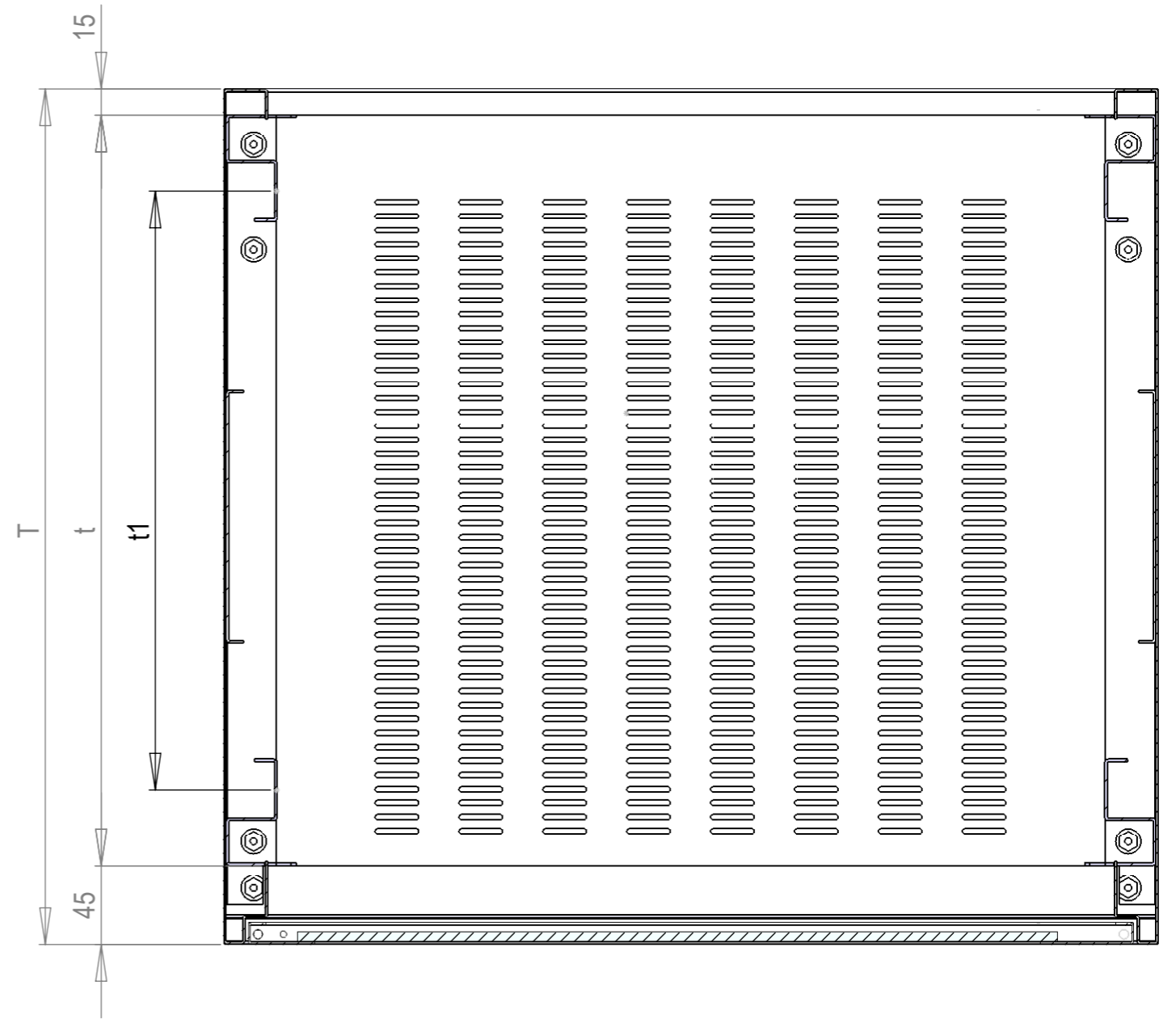
SCHNITT A-A
